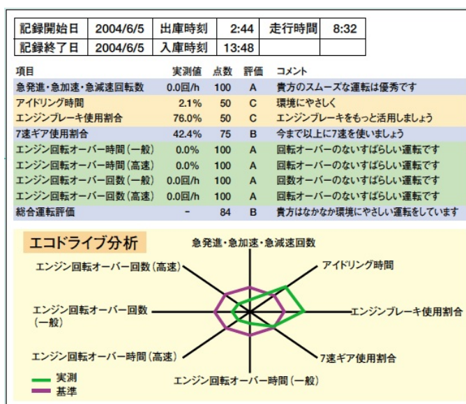
図 7.10 エコドライブ支援装置の概要とアウトプットの一例
