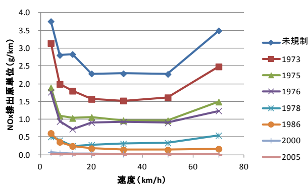
図 4.5 ガソリン・LPG 乗用車（４サイクル）の規制・車両総重量別の NO x 排出原単位の一例 (出所) 数理計画 自動車排出ガス原単位及び総量算定検討調査（2008）
